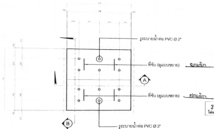
แบบขยายฝาปิดน้ำ ไม่แสดงมาตราส่วน
