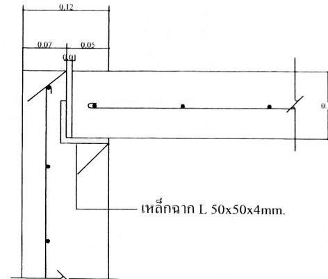
รูปขยายขอบวาง มาตราส่วน ไม่มี
