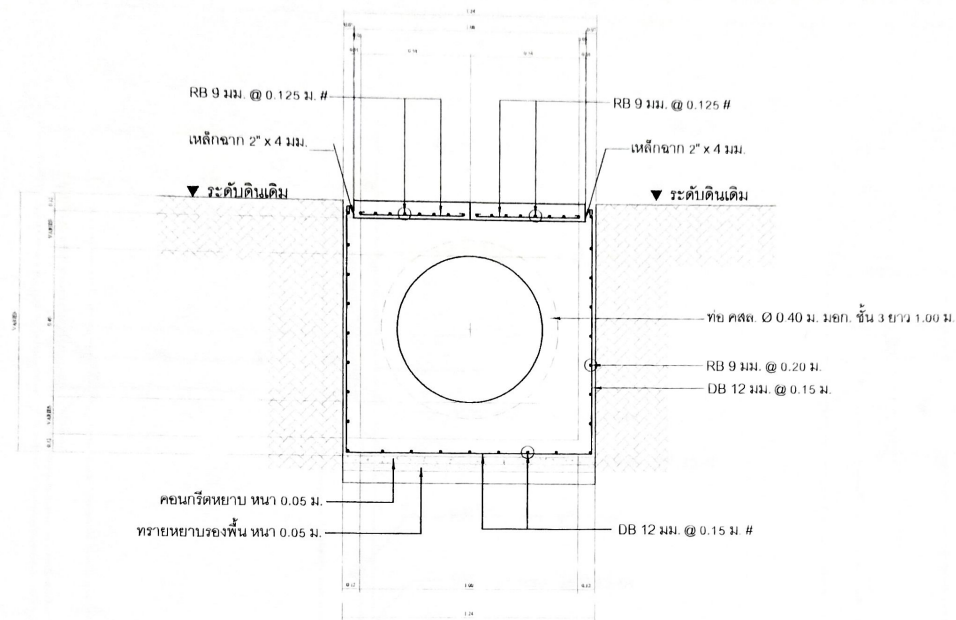
รูปตัด 2-2
