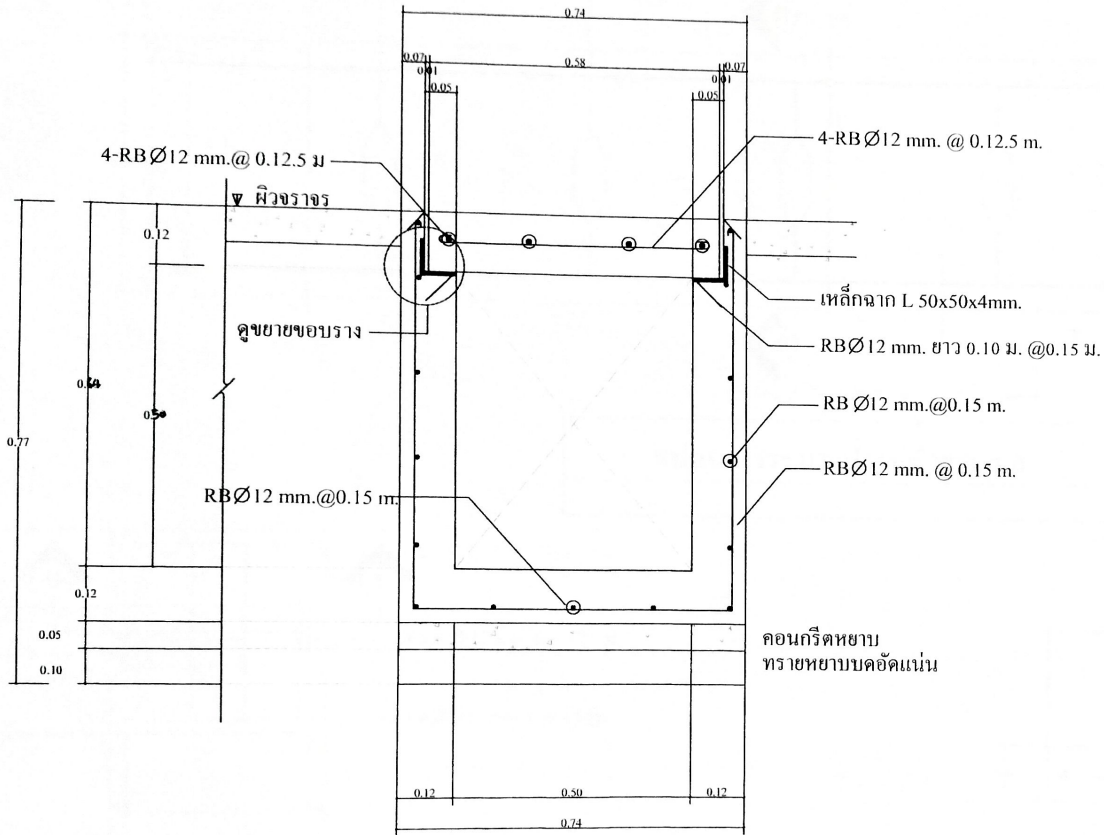
รูปตัด ก-ก มาตราส่วน ไม่มี
