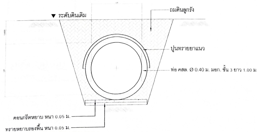
รูปตัด 3-3
